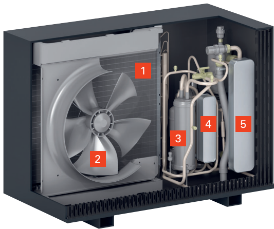
Außeneinheit: 2,1 bis 8,0 kW (A7/W35)
